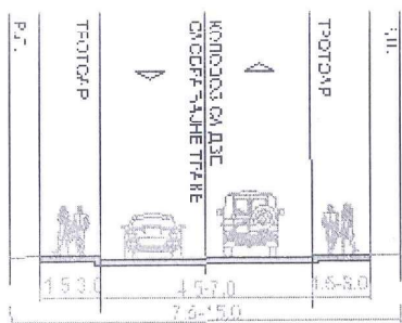
ПРОФИЛ 2-2 вар.1
