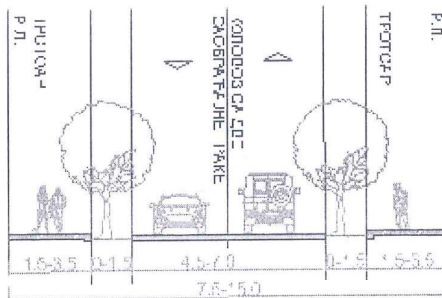
ПРОФИЛ 2-2 вар.2
